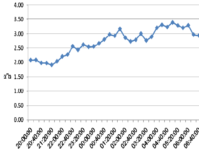
איור 1: ממוצע הפרש טמפרטורות אויר בין מבנה ללא מסך תרמי (חממה 5) לבין חממה עם מסך תרמי (חממה 2) ממוצע לתקופה של 15 ימים בין 15/1 ל15/2 בין השעה 20 00 ל7 00
